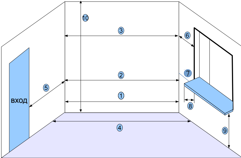
План-схема кухни
